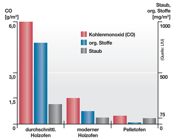
Vergleich der Schadstoffkonzentrationen im Abgas von Holzöfen
