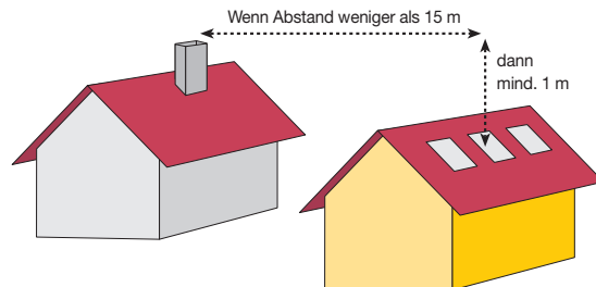
Mindesthöhe von Kaminmündungen in Abhängigkeit der Entfernung zum benachbarten Wohngebäude.
